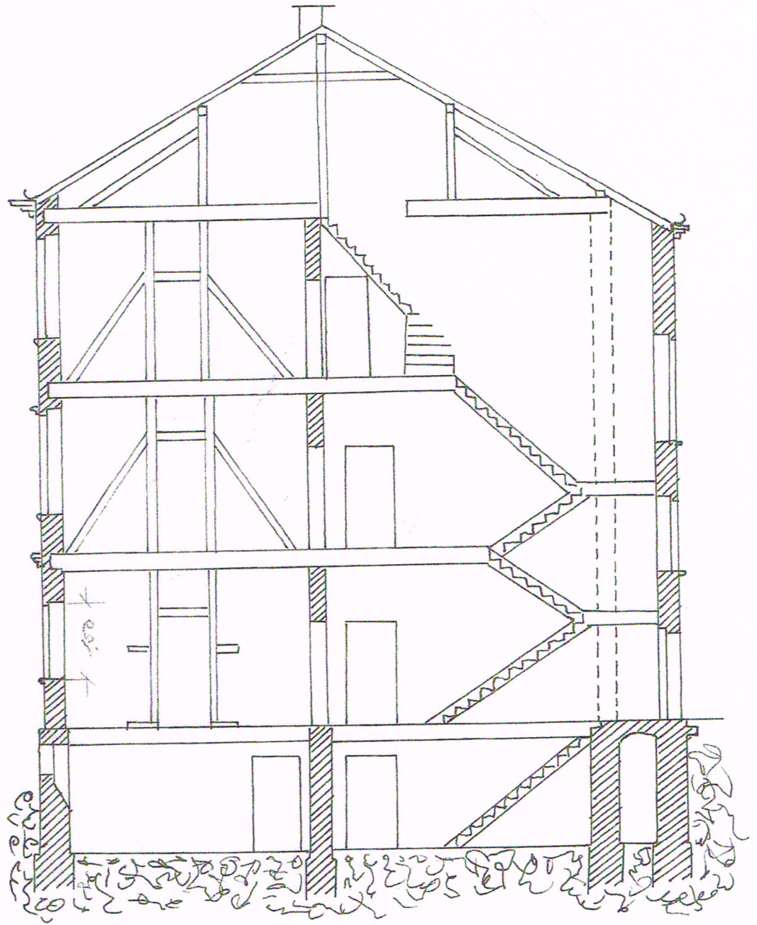
Querschnitt
